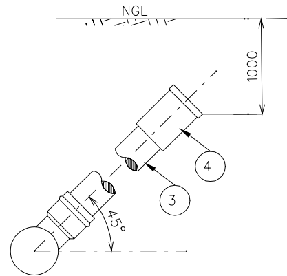
TYPICAL ELEVATION RAMP RISER N.T.S.
