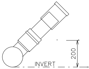
TYPICAL ELEVATION NO RAMP RISER N.T.S.
