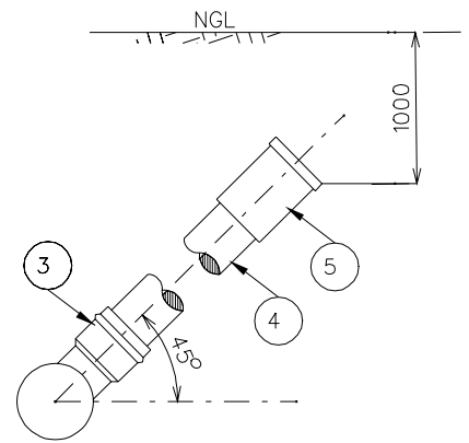
TYPICAL ELEVATION RAMP RISER N.T.S.
