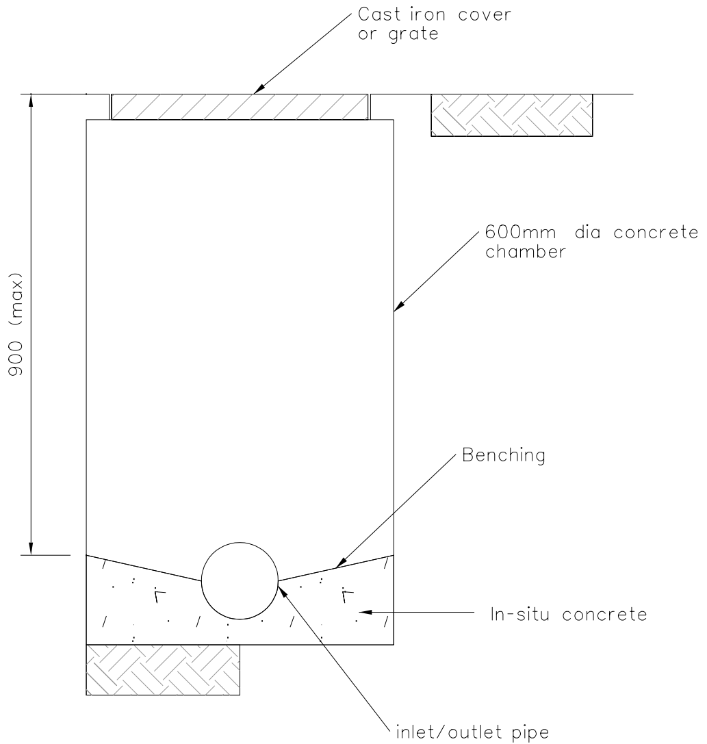
MINI MANHOLE SECTIONAL ELEVATION
